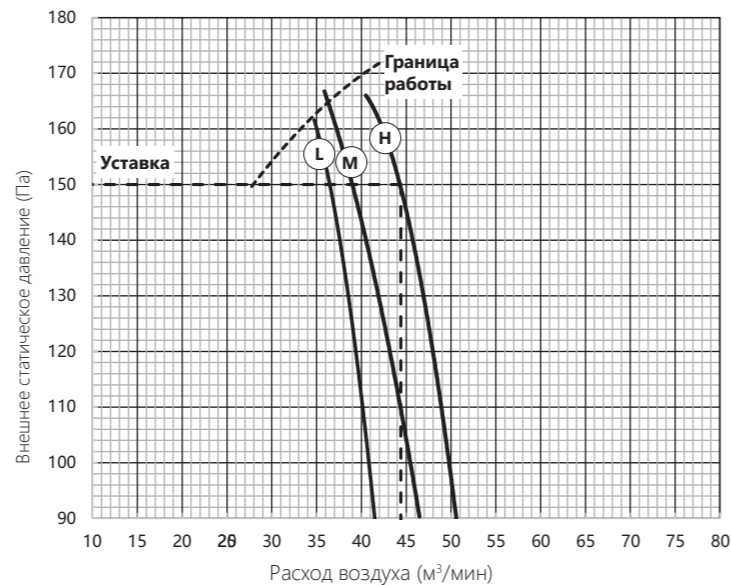
AUD-48HX4REM2/AUD-60HX4REM2(уставка 150 Па)
