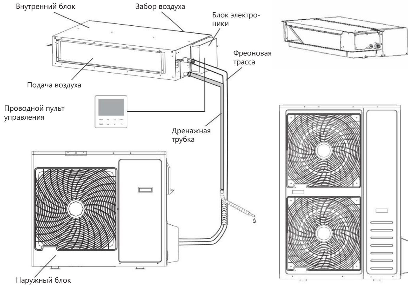
Наружный блок (типоразмер 12/18/24/36)
