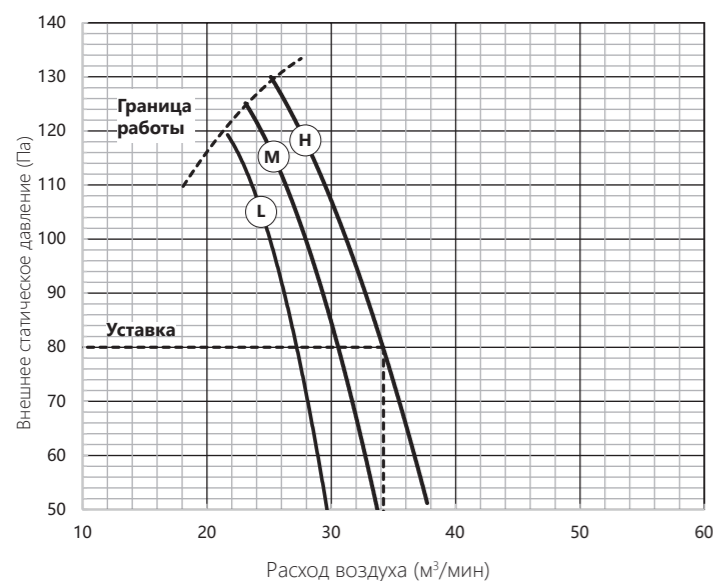
AUD-48HX4REM2/AUD-60HX4REM2 (уставка 80 Па)
