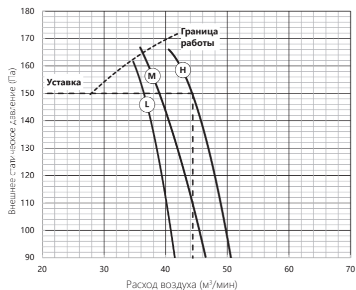
AUD-48HX4REM2/AUD-60HX4REM2(уставка 150 Па)
