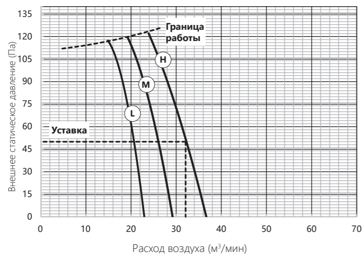
AUD-36HX4RFM2(уставка 60 Па)
